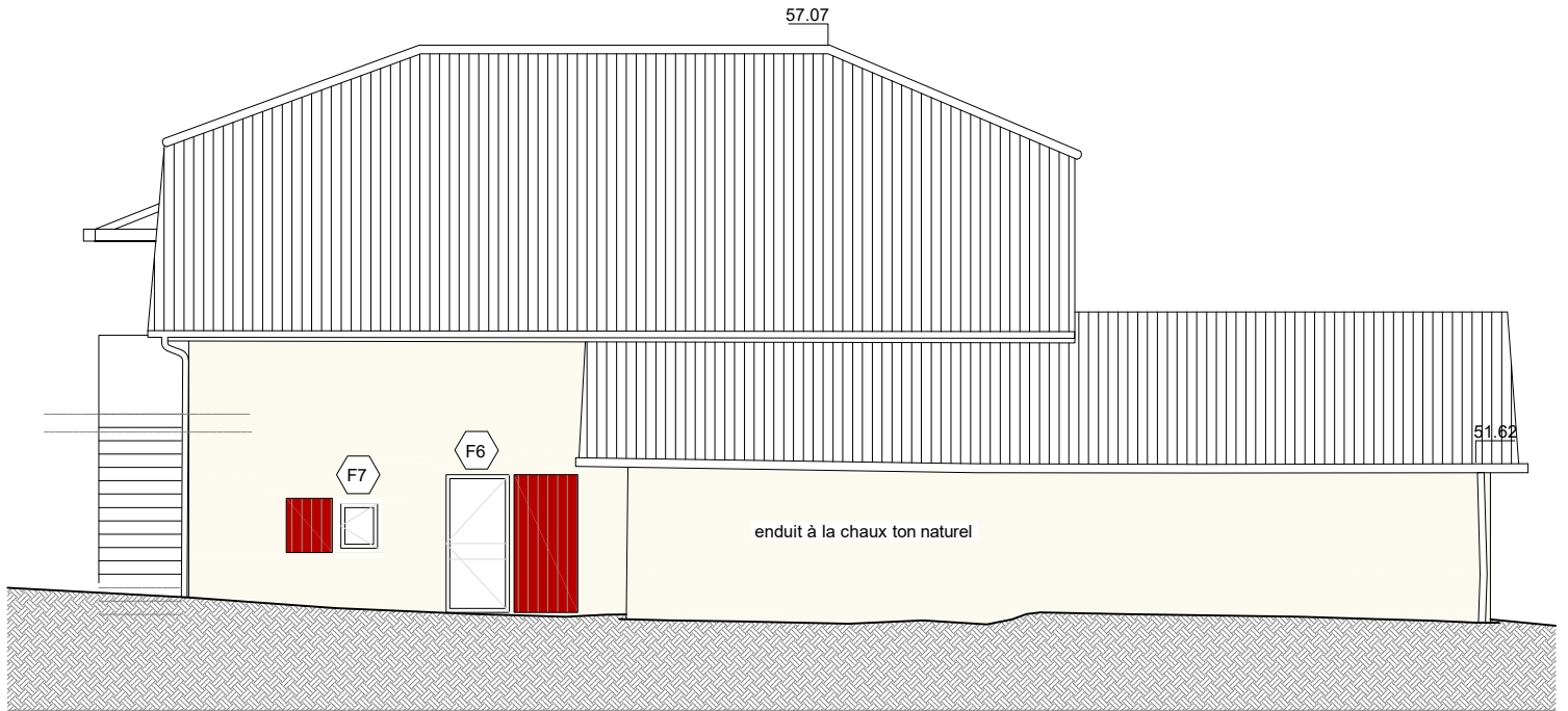
FACADE NORD
